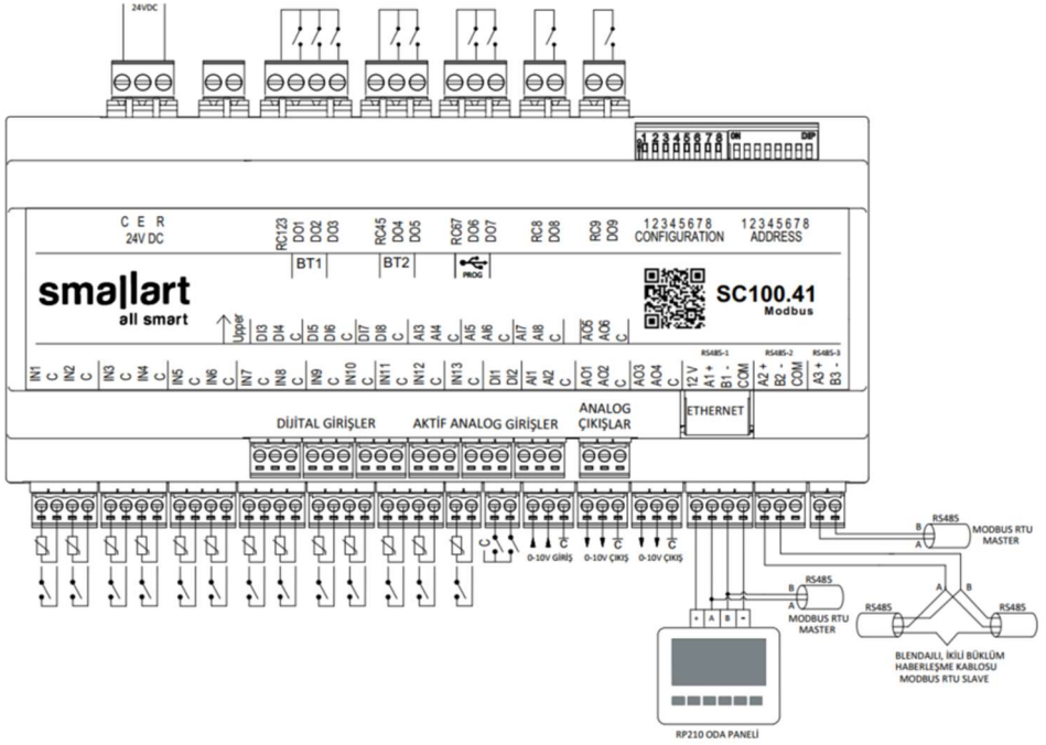
SC100 Bağlantı Şeması
