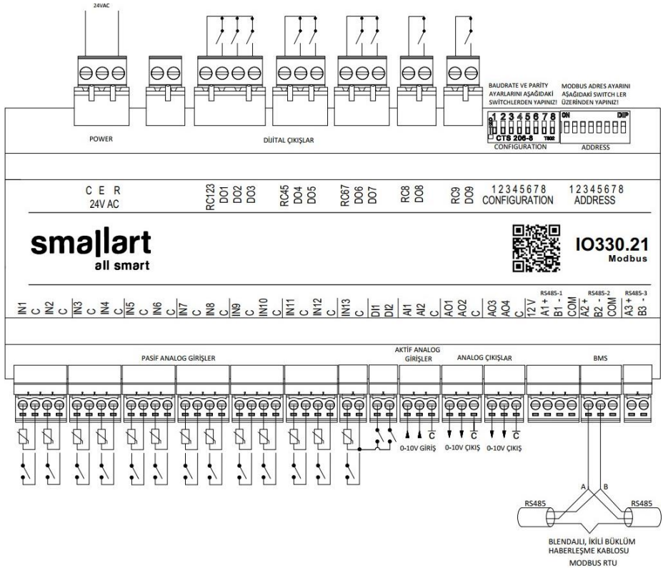
IO330.21 Bağlantı Şeması
