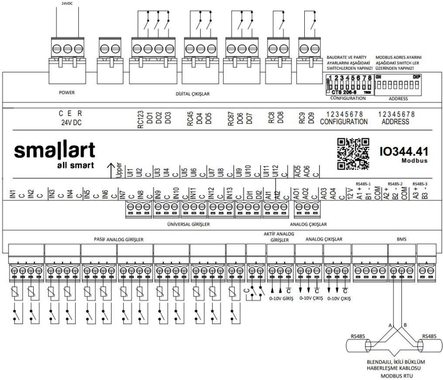
IO344.41 Bağlantı Şeması
