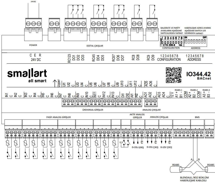
IO344 Bağlantı Şeması
