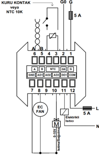
2 Borulu Fan Coil ve 6-Yollu Vana için Bağlantı Şeması
