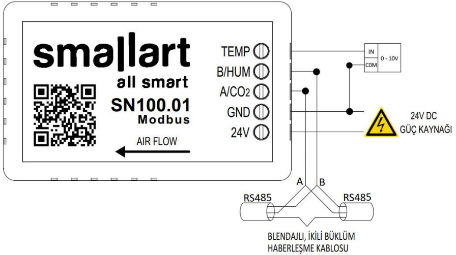
SN100 Bağlantı Şeması (1 Adet 0-10V Analog Çıkışı ve RS485 Haberleşme)
