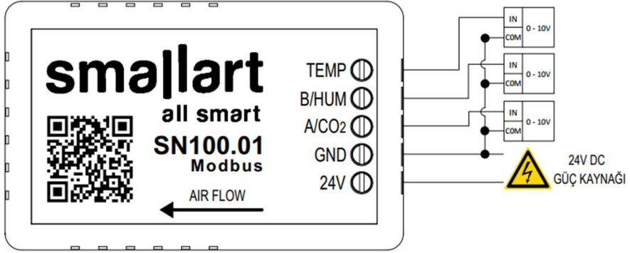
SN100 Bağlantı Şeması (3 Adet 0-10V Analog Çıkışı)
